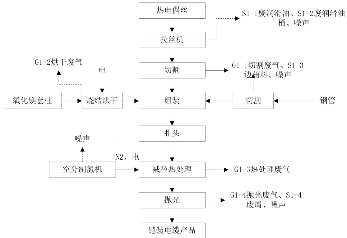
图 2.2-2 铠装电缆工艺流程及产排污环节
