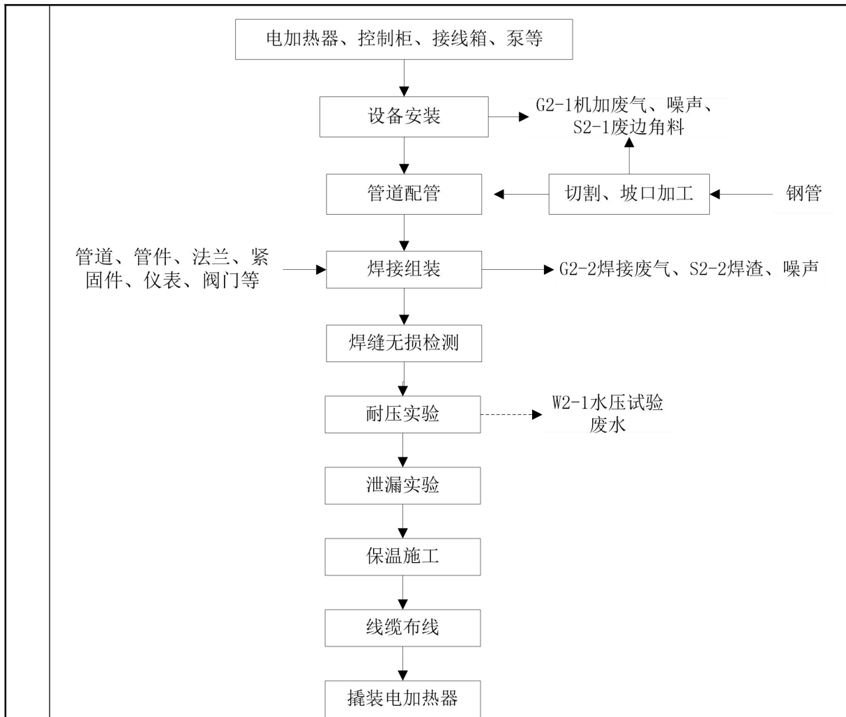
图 2.2-3 撬装电加热器生产工艺流程及产排污环节
