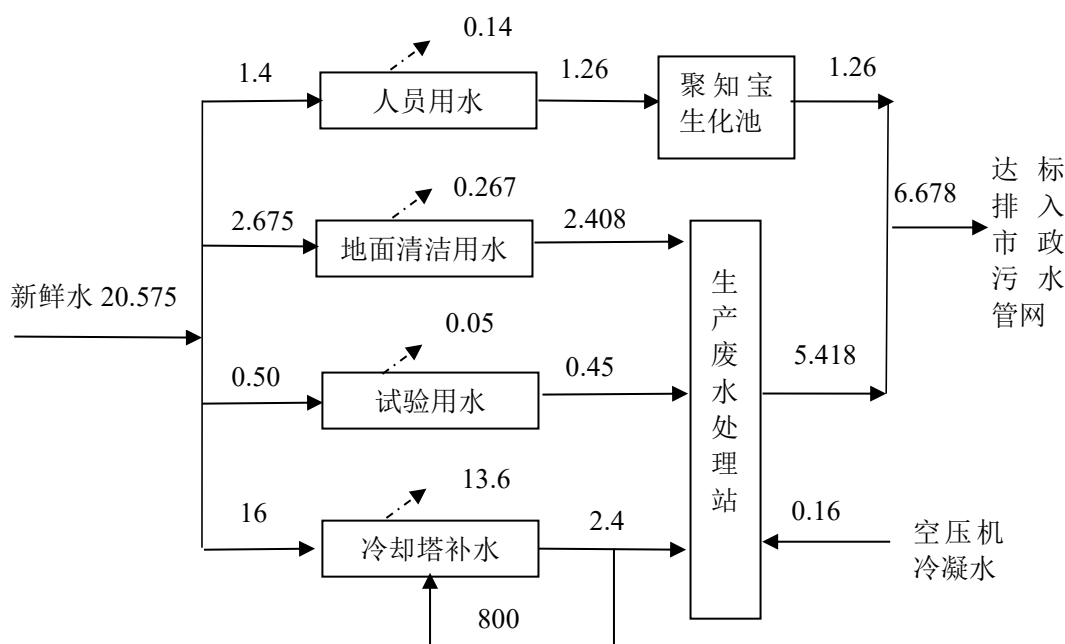
图 2.1-1 本项目水平衡图 单位: m 3 /d
